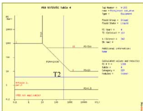
Slika 2b: Dijagrami za određivanje kategorije OPP - na strani tople vode (tačka T2)
