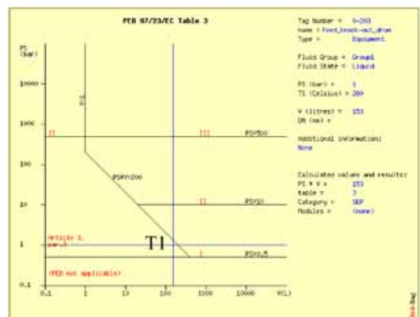
Slika 2a: Dijagrami za određivanje kategorije OPP - na strani termo ulja (tačka T1)
